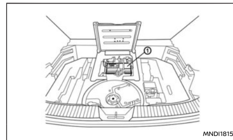
Exemple d'emplacement de la batterie 12 V
