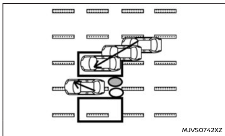
Illustration 10 Entrée latérale dans le périmètre de détection
