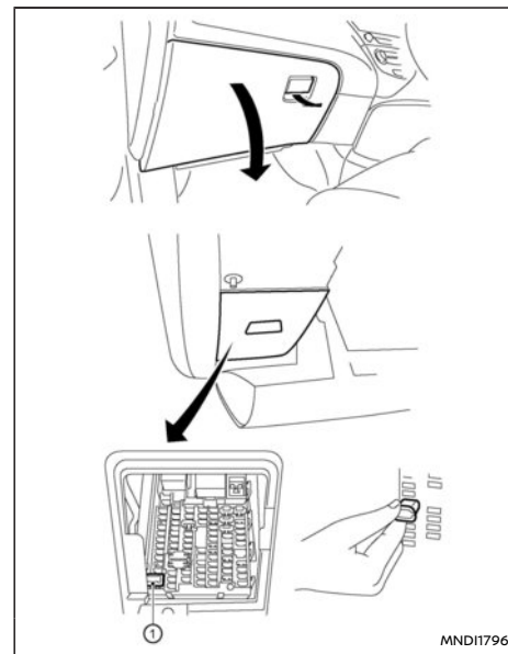
Boîte à fusibles principale, modèles à conduite à droite
