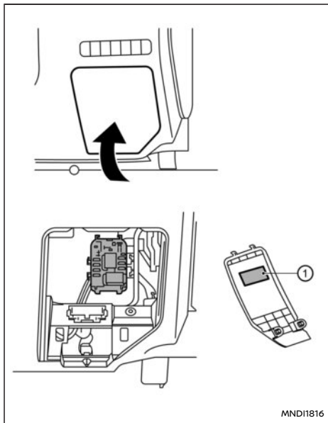
Boîte à fusibles secondaire, modèles à conduite à droite
