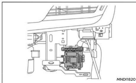
Boîte à fusibles secondaire, modèles à conduite à gauche
