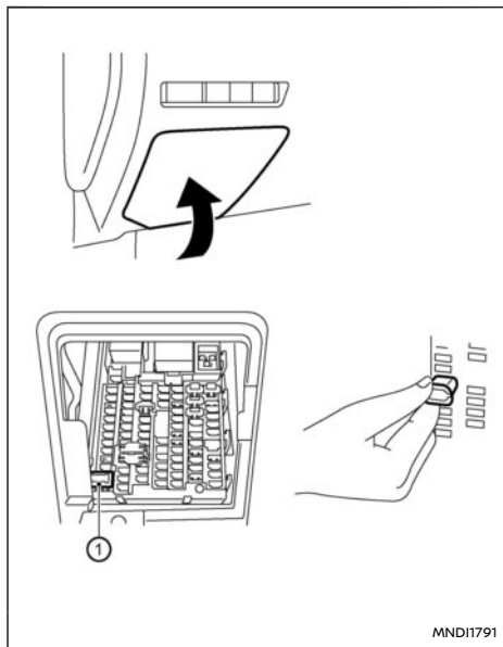
Boîte à fusibles principale, modèles à conduite à gauche
